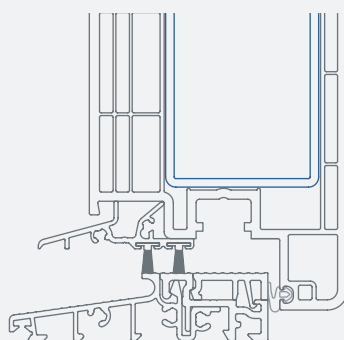
Drzwi otwierane do wewnątrz
