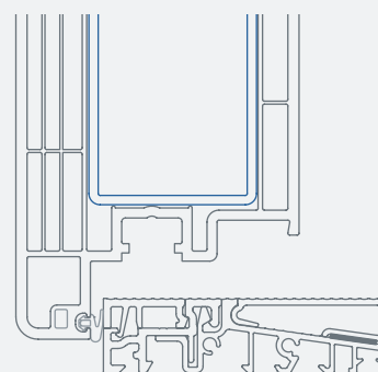
Drzwi otwierane na zewnątrz
