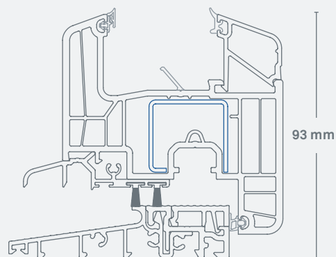
Nowość : Bezbarierowy próg do drzwi balkonowych Rys.: 1:2
